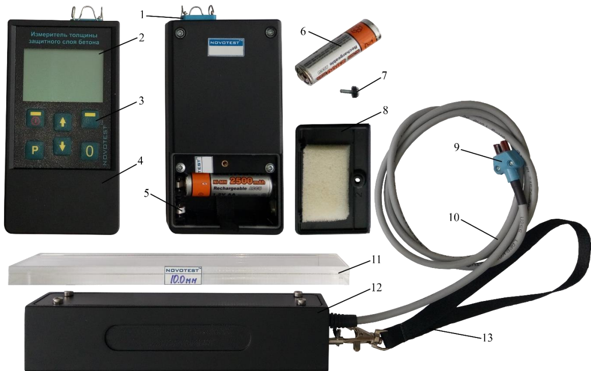
1 – разъем подключения преобразователя; 2 – графический индикатор (дисплей); 3 – клавиатура управления; 4 – корпус; 5 – батарейный отсек; 6 – аккумуляторная батарея; 7 – винт фиксации крышки батарейного отсека; 8 – крышка батарейного отсека; 9 – штекер подключения преобразователя; 10 – кабель преобразователя; 11 – диэлектрическая прокладка; 12 – преобразователь; 13 – ремень фиксации преобразователя.
